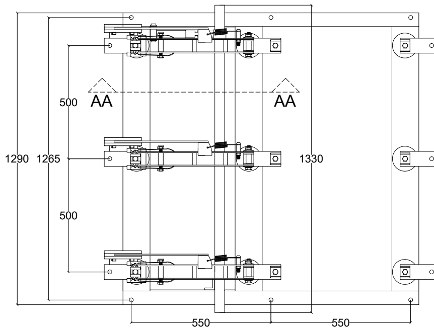
CORTE AA
